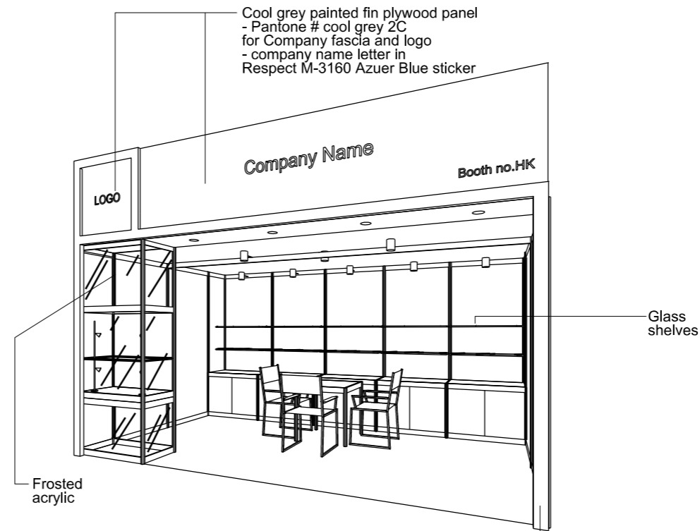
PERSPECTIVE N.T.S.
