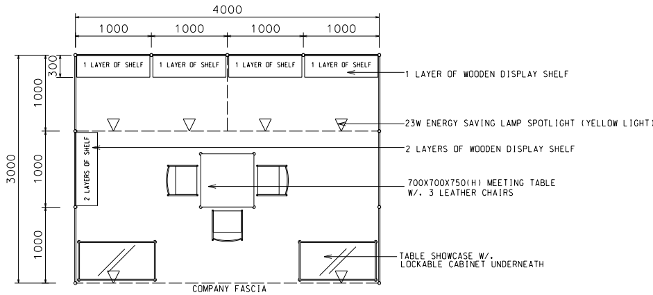
PLAN 平面圖
