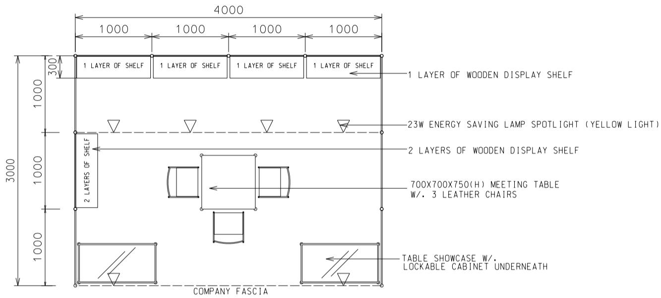
PLAN 平面圖
